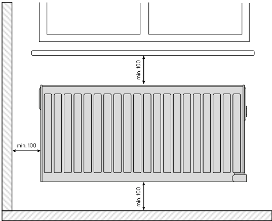
Yali - min afstanden bevestiging
